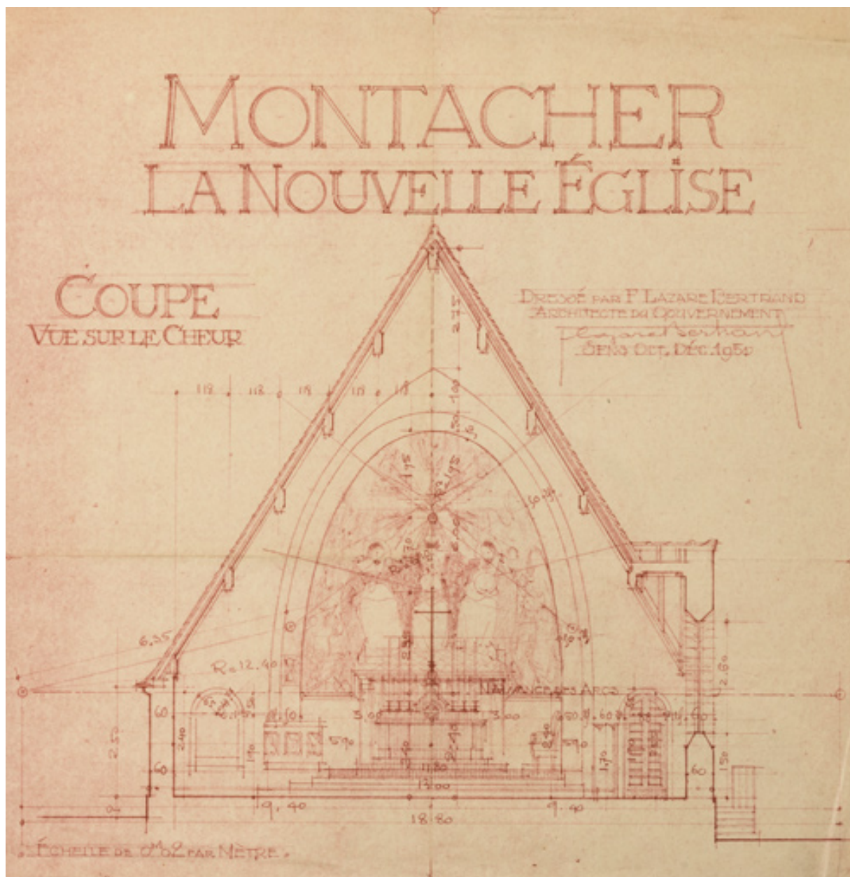
Coupe transversale : vue sur le chœur, 1950.
