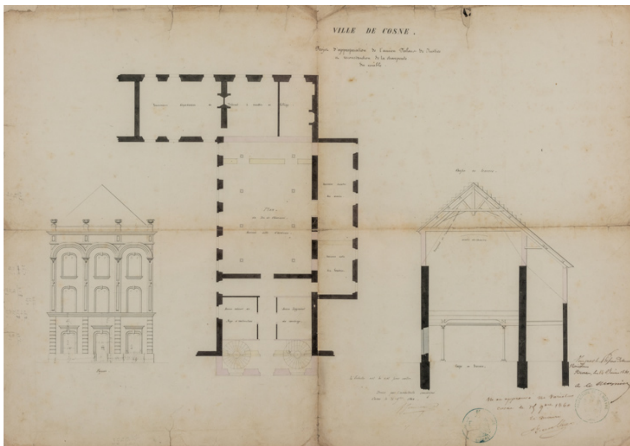
Ville de Cosne. Projet d'appropriation de l'ancien palais de justice et reconstruction de la charpente du comble. 15 novembre 1860.
