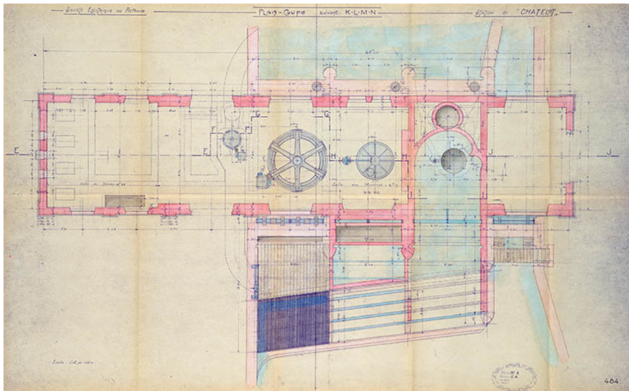
Société Electrique de Belchamp. Station du Chatelot. Plan-coupe de l'usine, pièce n° 9, 1934.
