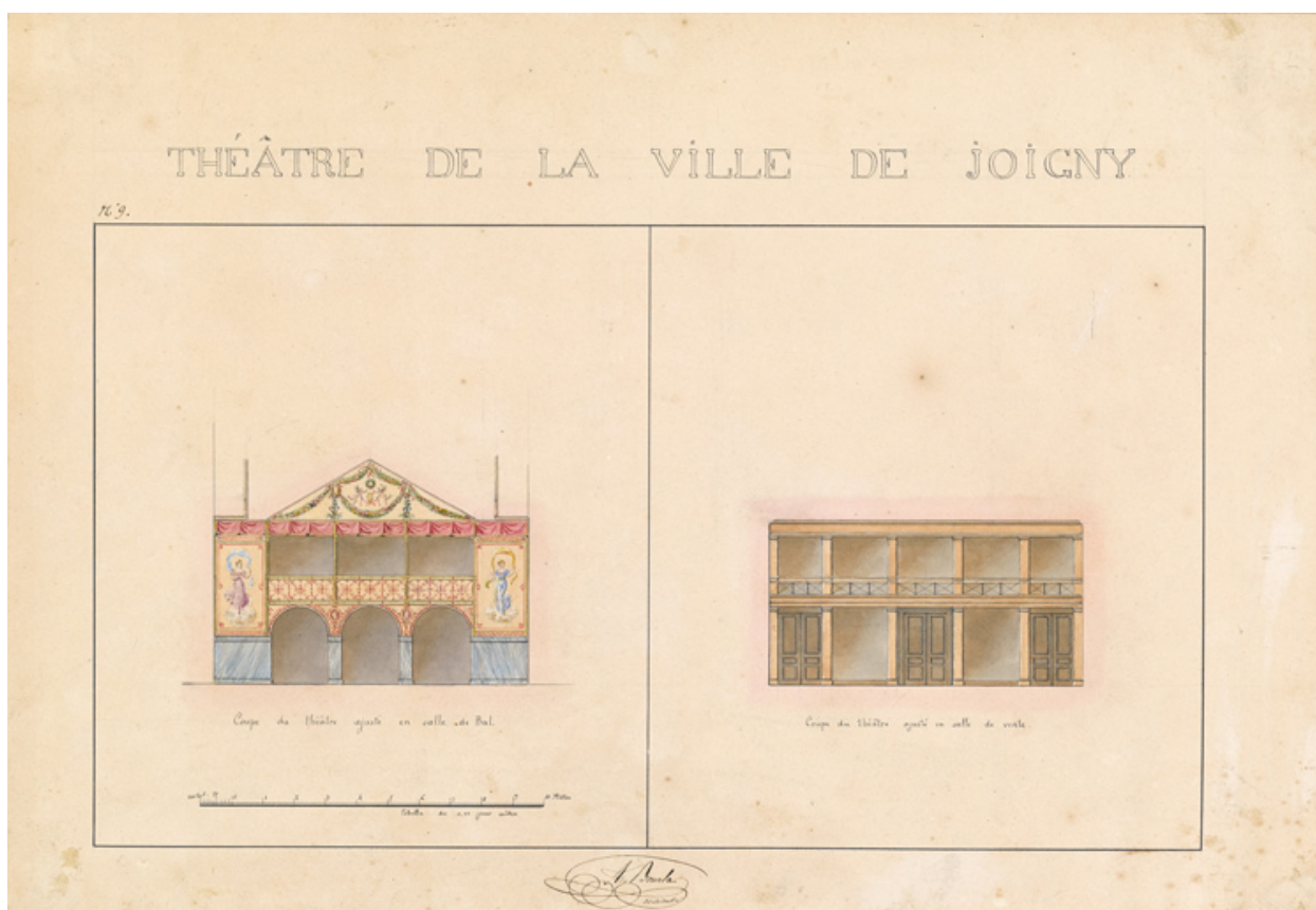
Coupe du théâtre ajusté en salle de bal [et] Coupe du théâtre ajusté en salle de vente. N° 9. S.d. [1829-1830]. (MAP : G/82/89/2008-039061)
