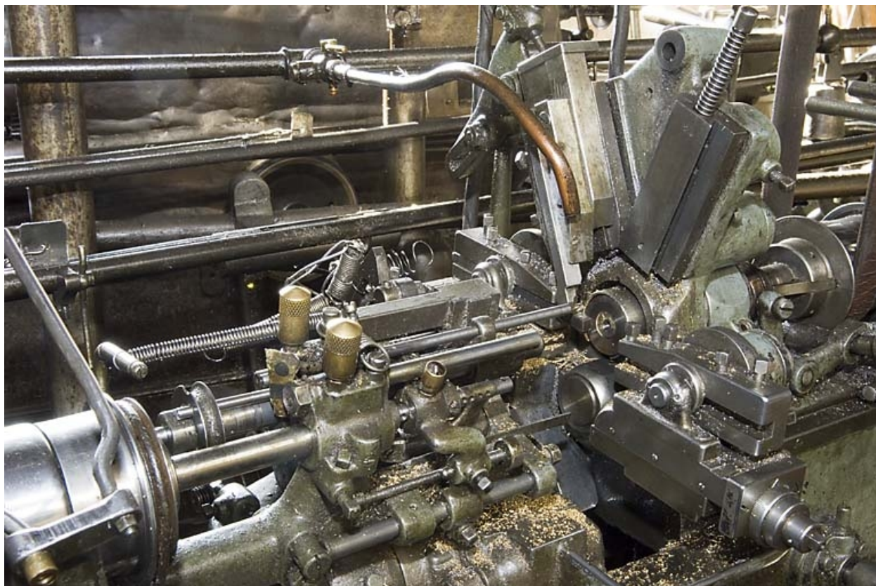
Détail des outils de coupe d'un tour à décolleter Petermann (M).
