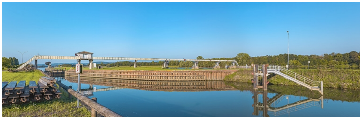
Tête amont de l'écluse.
