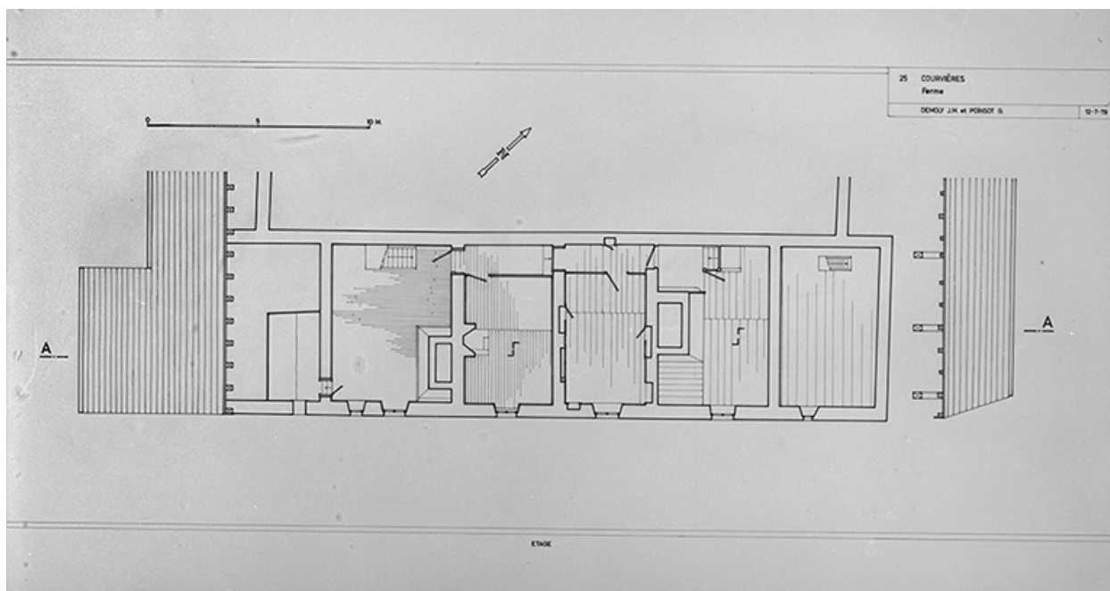
Plan du 1er étage, partie habitation d'une ferme..
