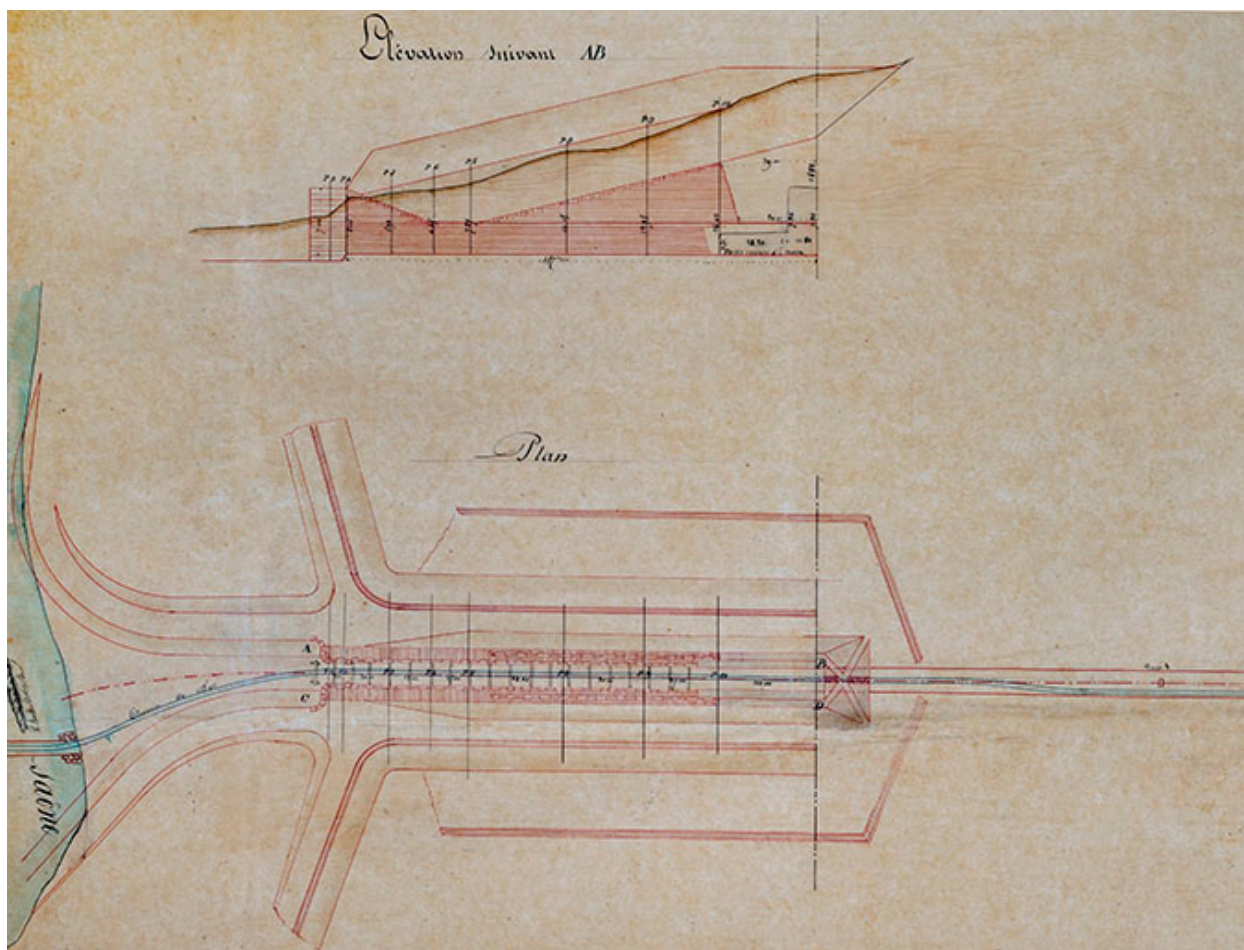
Plans et profils de la dérivation souterraine de Saint-Albin, 1843 : partie amont.
