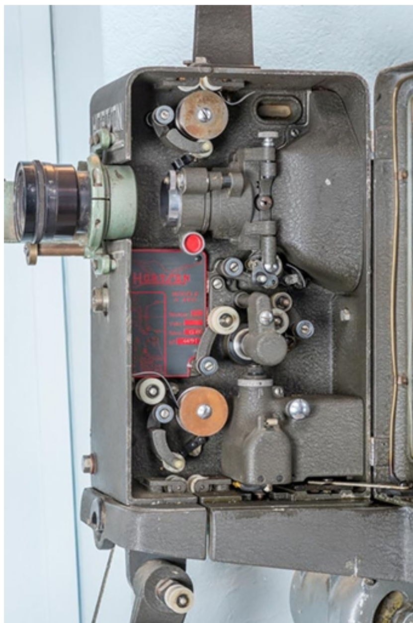
Mécanisme projecteur (système d'entraînement du film et objectif).
