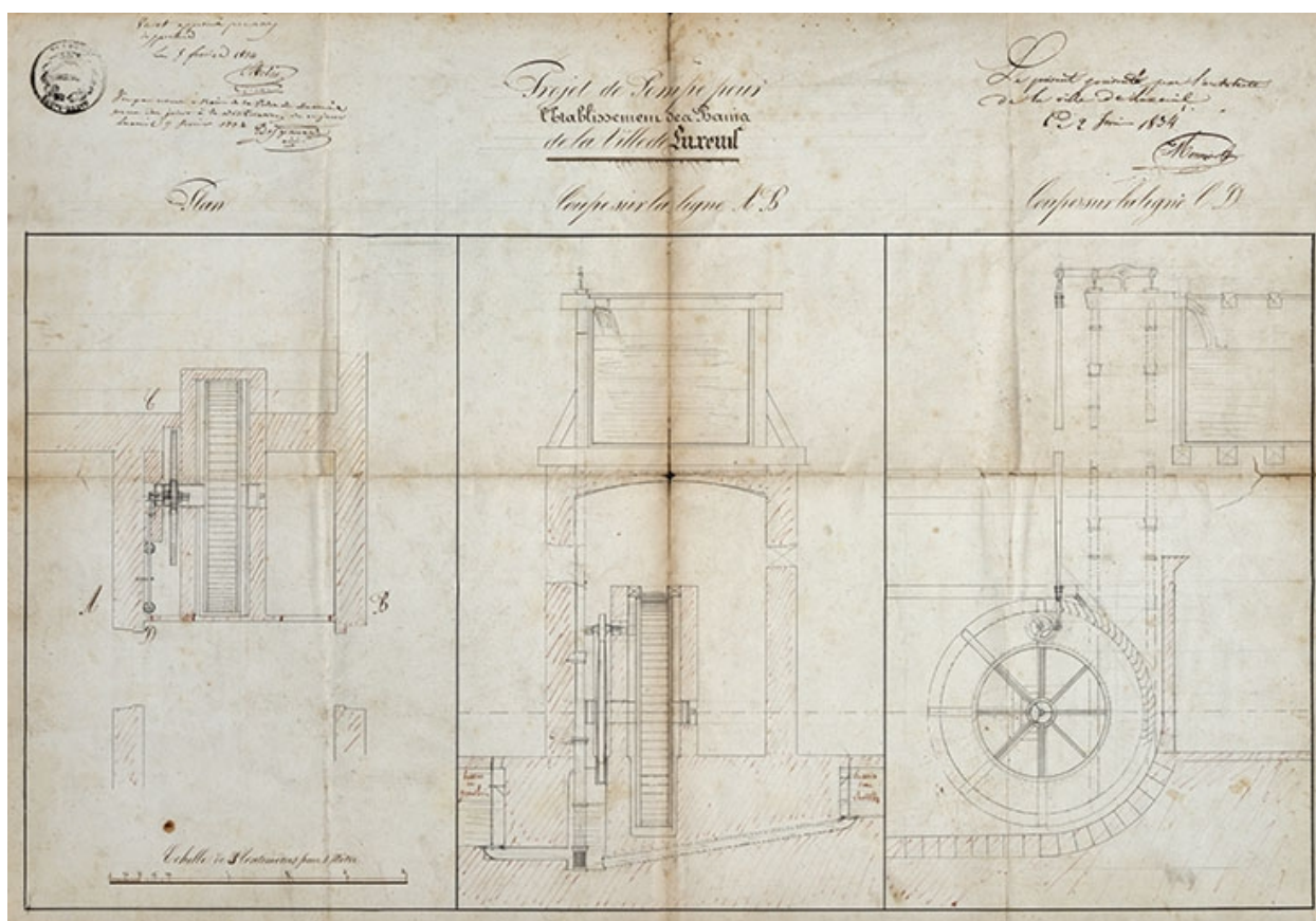
Projet de pompe (2 février 1834).
