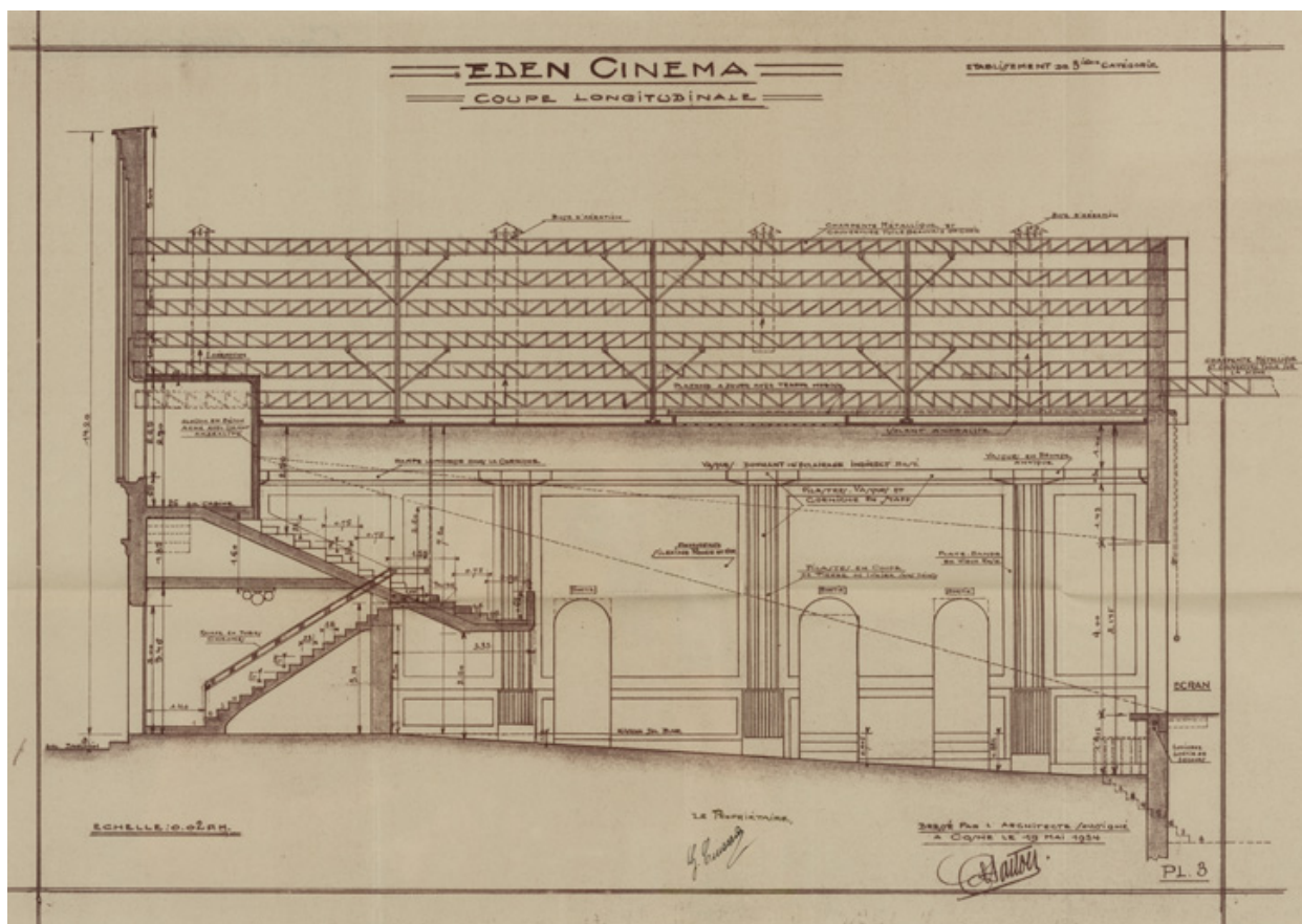
Eden-Cinéma. Coupe longitudinale. 1934.
