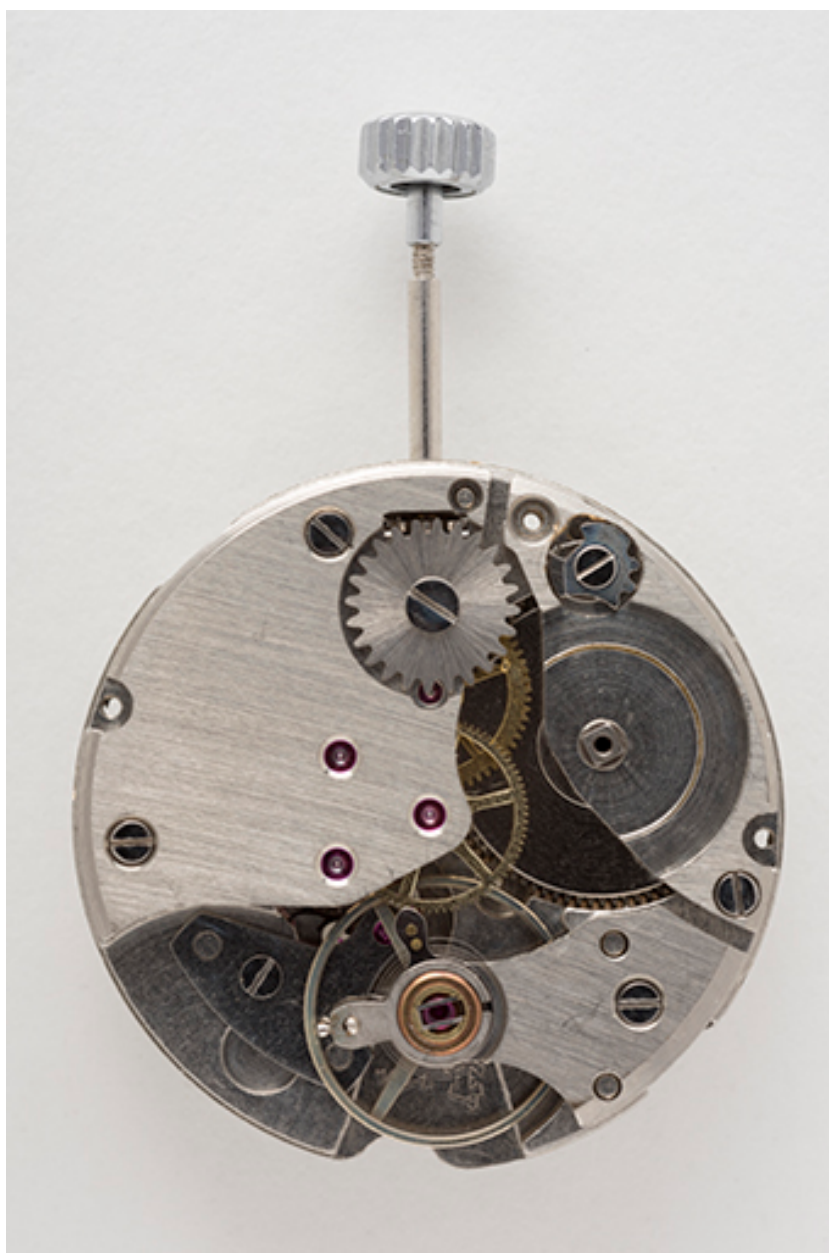
Mouvement FE 140-1, vu côté pont.
