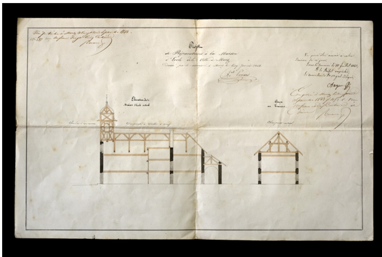
Projet de réparations à la maison d'école de la ville de Morez. Elévation de la maison d'école actuel [et] Coupe en travers, 1843.
