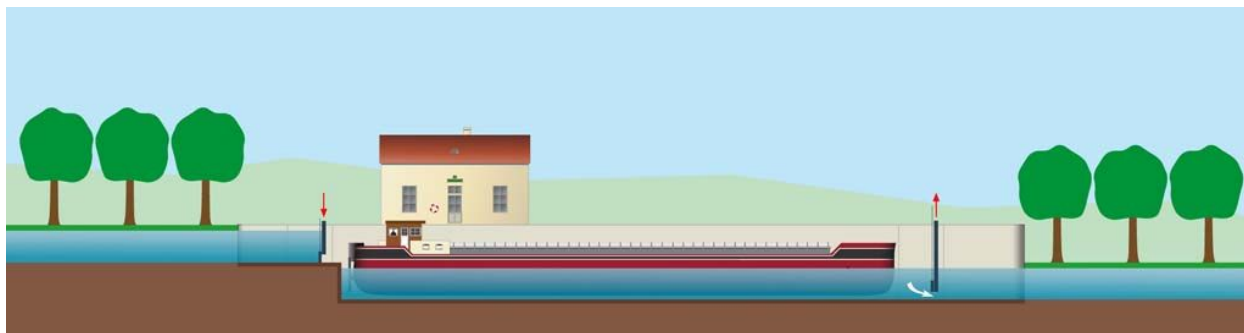
Schéma d'éclusement d'un bateau avalant, étape 7.
