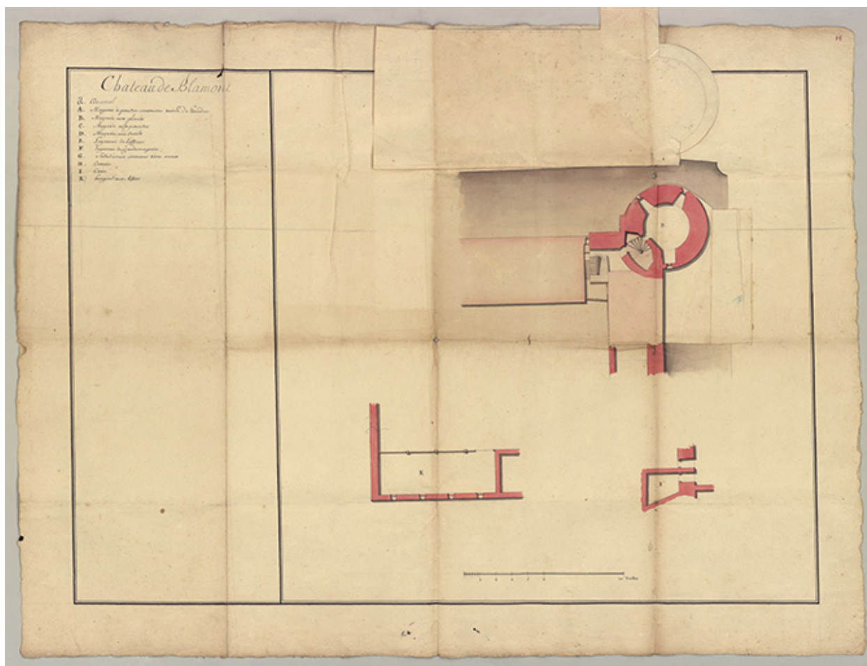
Fol. 18 Château de Blamont : plans (magasin pour 10,000 milliers de poudre) [vue 3].
