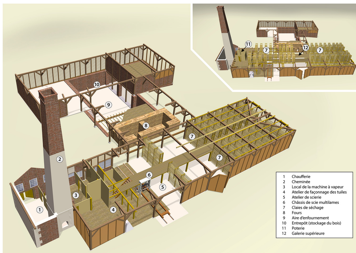
Vue axonométrique de la tuilerie-scierie des Combes de Punay (Malbrans).
