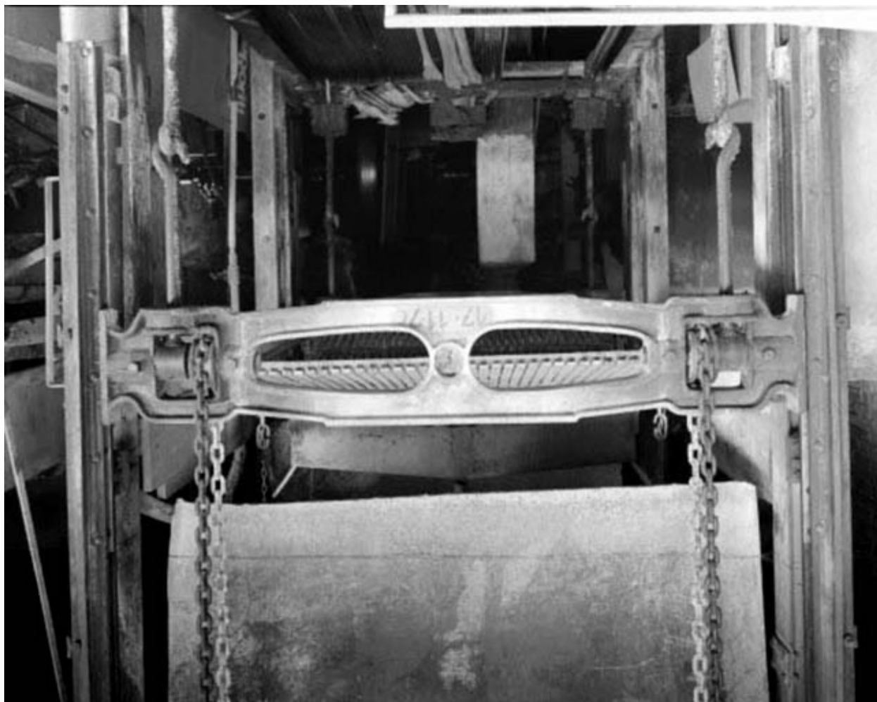
Guide support d'un châssis porte-lames.
