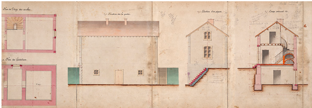
Construction de la dérivation de Port-sur-Saône - Maison éclusière (1876).
