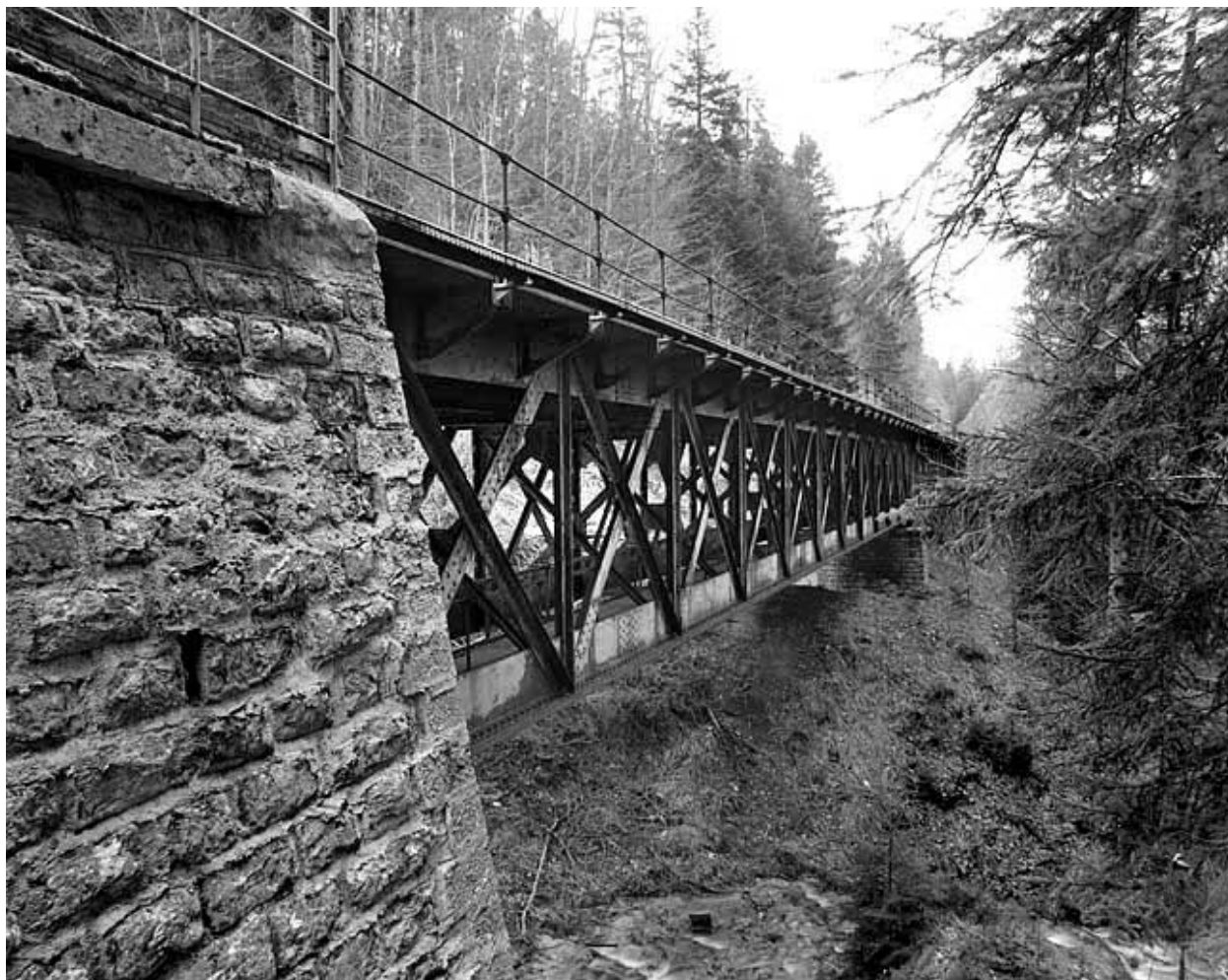
Viaduc de la Renvoise (Chaux-des-Crotenay) : vue d'ensemble en enfilade, depuis le côté La Cluse.
