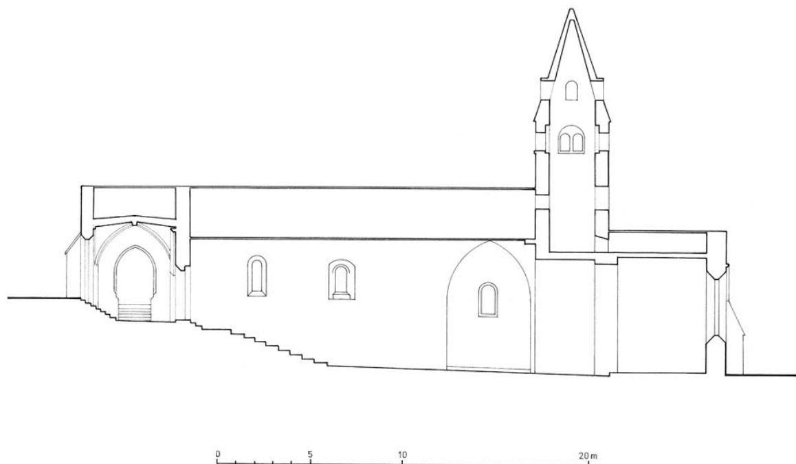
coupe longitudinale
