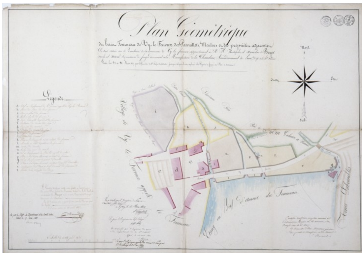
Plan géométrique du haut fourneau de Vy-le-Ferroux, des patouillets, moulins [...].
