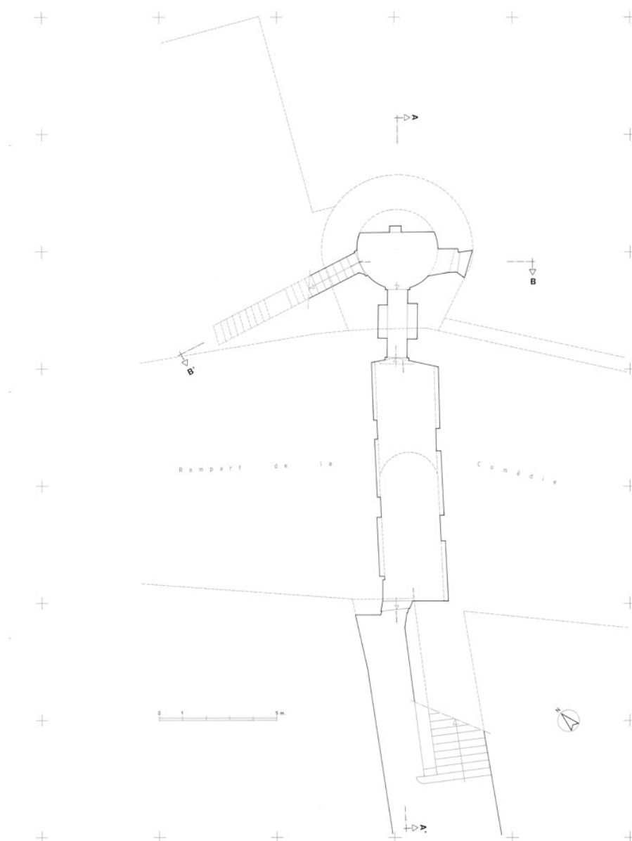
Tour Notre-Dame. Plan du niveau inférieur.
