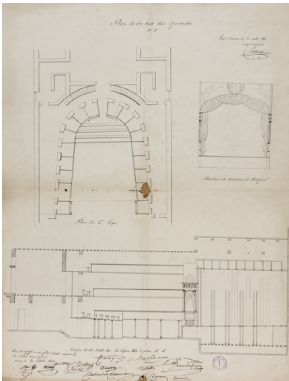
Plan de la salle des spectacles. N° 2. Plan des 1ères loges, Coupe de la salle sur la ligne AB du plan N° 1er [et] Elévation du Manteau d'Arlequin. 23 octobre 1822.
