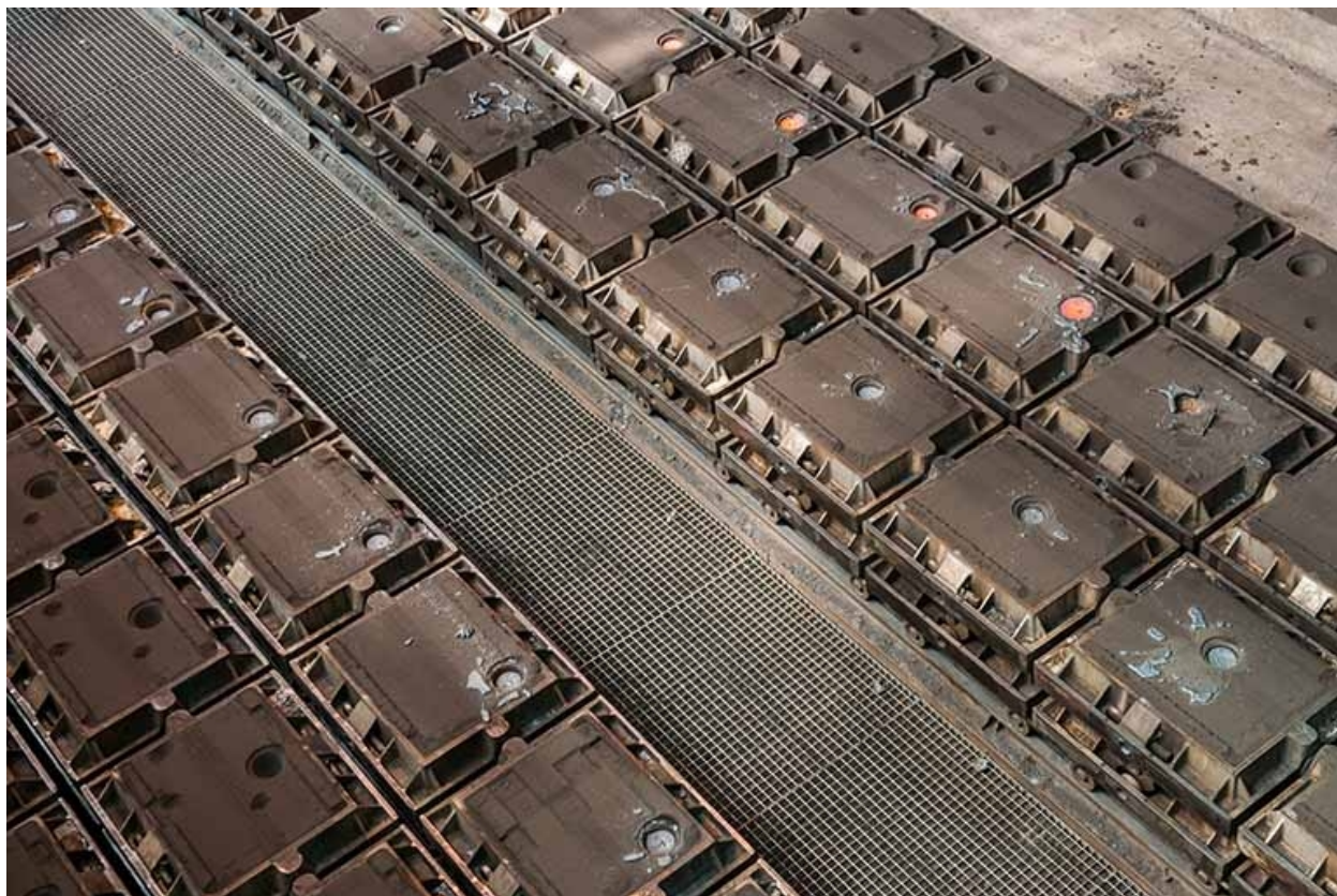
Ligne de moulage. Détail des moules (3).
