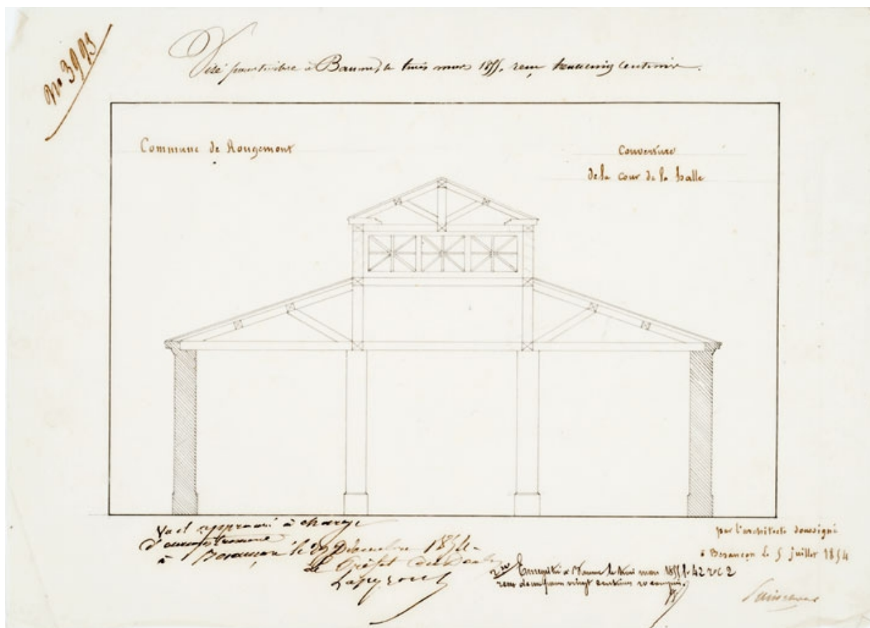
Commune de Rougemont. Couverture de la cour de la halle. 5 juillet 1854.
