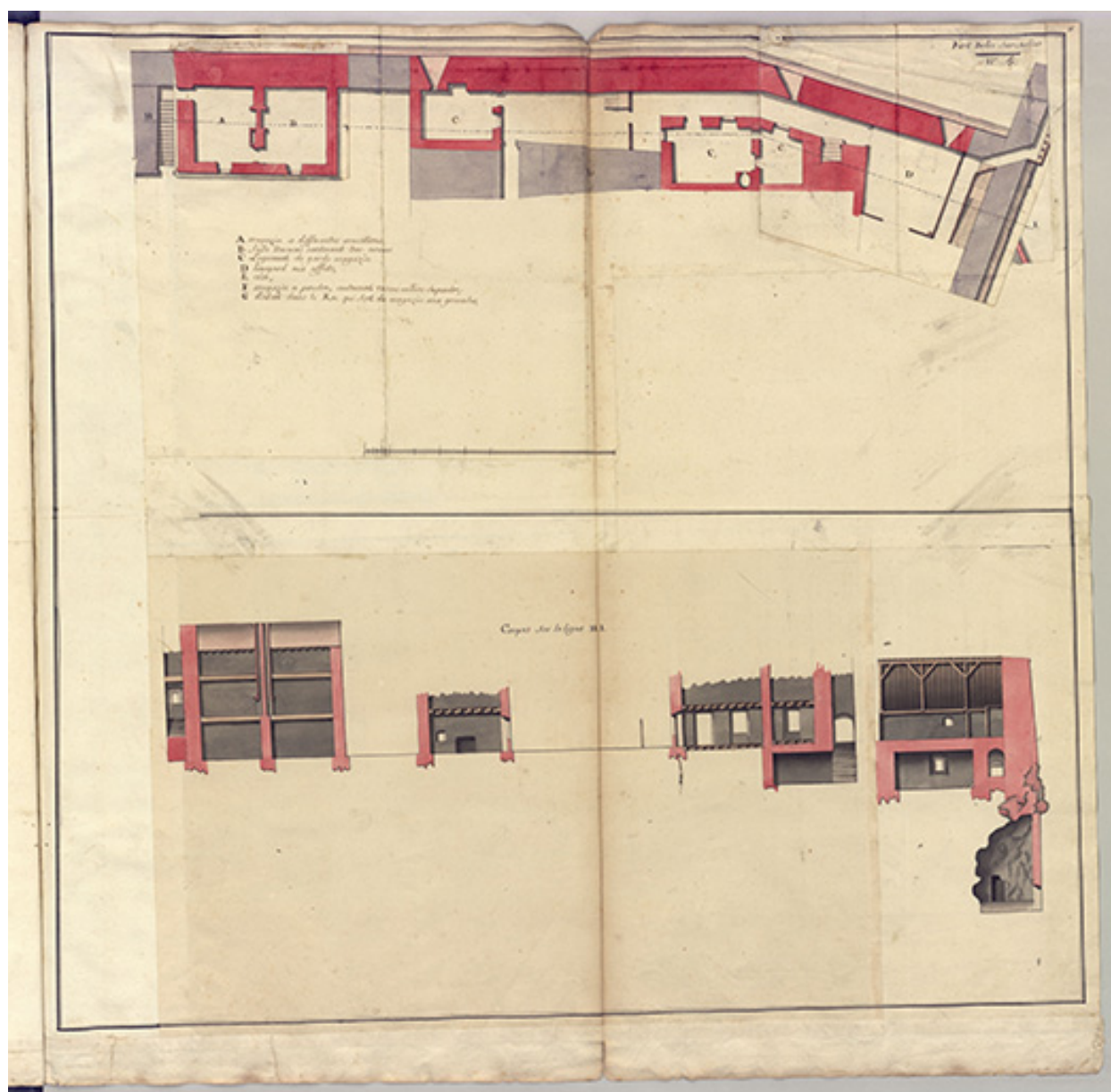
Fol. 16 Fort-Belin-sur-Salins : plans et coupes (magasin pour 12,000 milliers de poudre) - vue 1.
