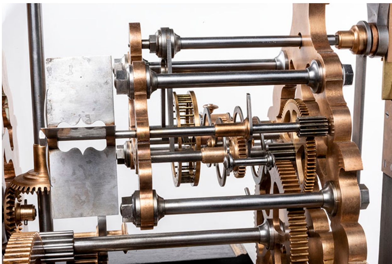
Mouvement : détail du mécanisme.
