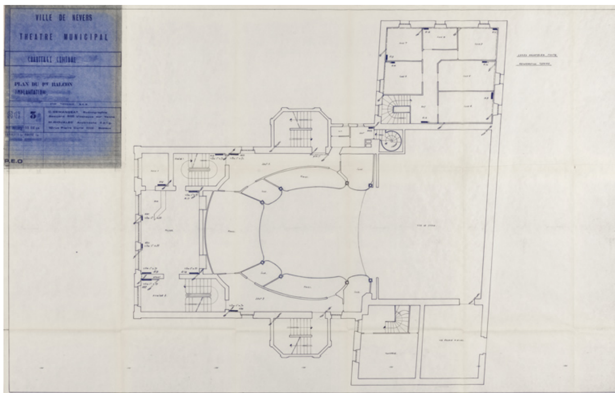
Ville de Nevers. Théâtre municipal. Chauffage central. SC 3. Implantation. Plan du 1er balcon. Octobre 1978.
