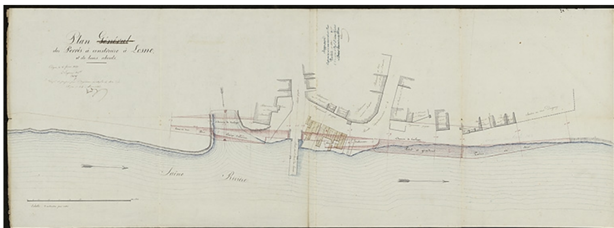
Plan des perrés à construire à Losne et de leurs abords. 1838.
