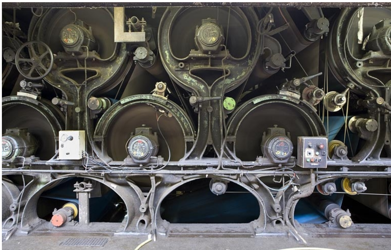
Fabrique de cellulose et usine à papier Jean-Baptiste Weibel et Cie, puis Otor-Papeterie du Doubs, Novillars : calandres de la machine à papier.
