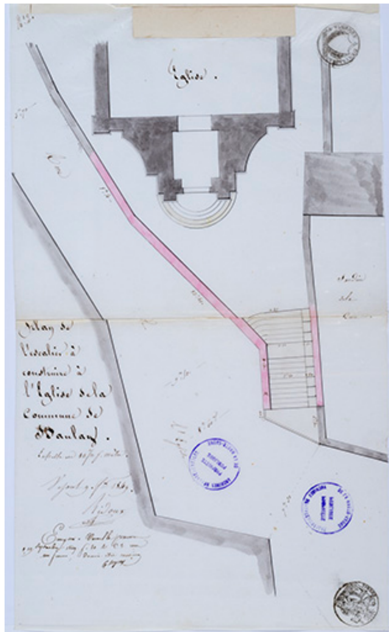
Plan du projet de construction d'un escalier permettant d'accéder au parvis de l'église, 1849
