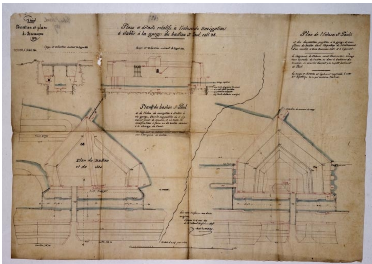
Plans et détails relatifs à l'écluse de navigation à établir à la gorge du bastion St Paul, coté 38 [plans, coupe et élévation], 1827.
