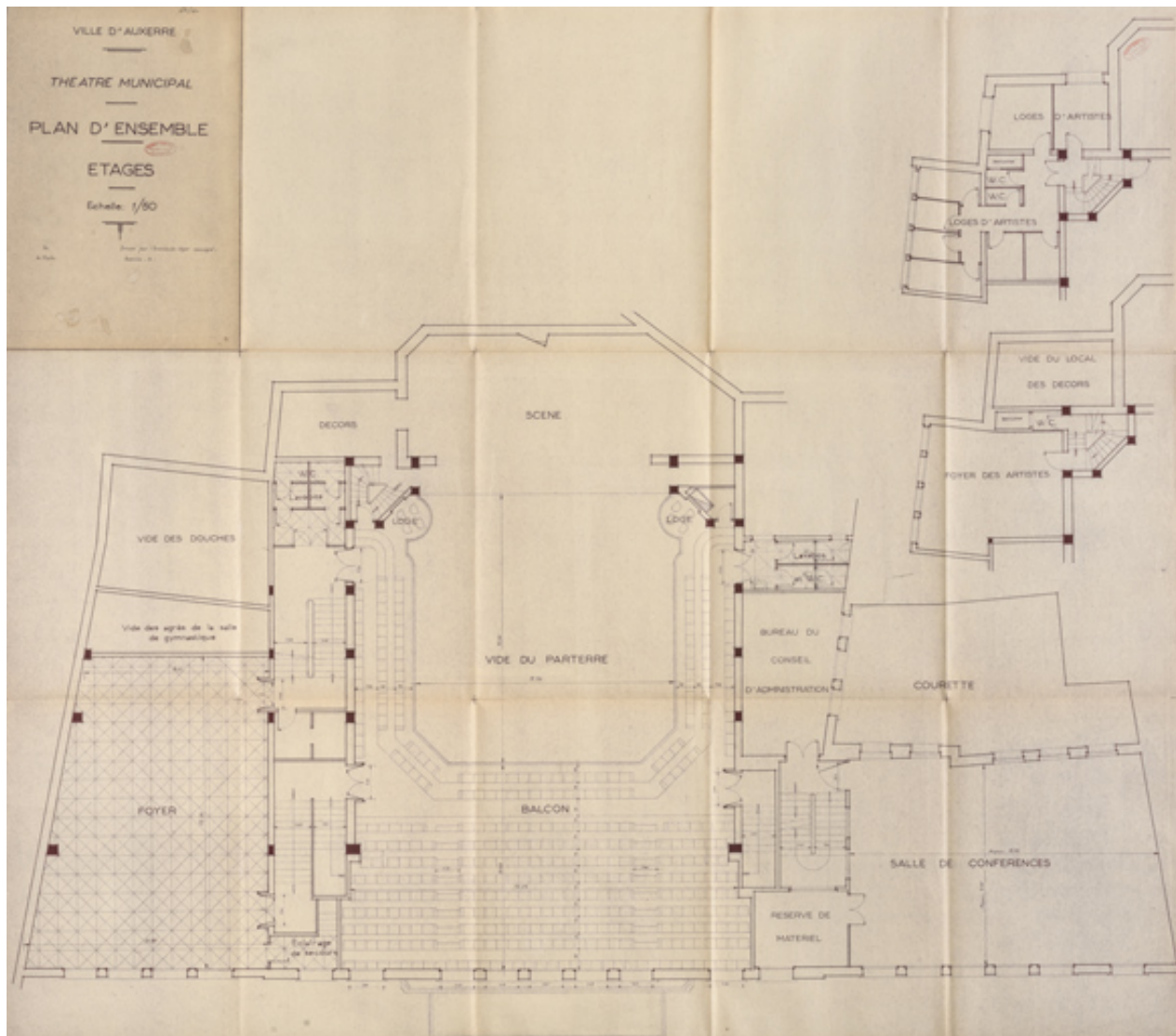
Ville d'Auxerre. Théâtre municipal [plans]. Etages. S.d. [1952 ?].
