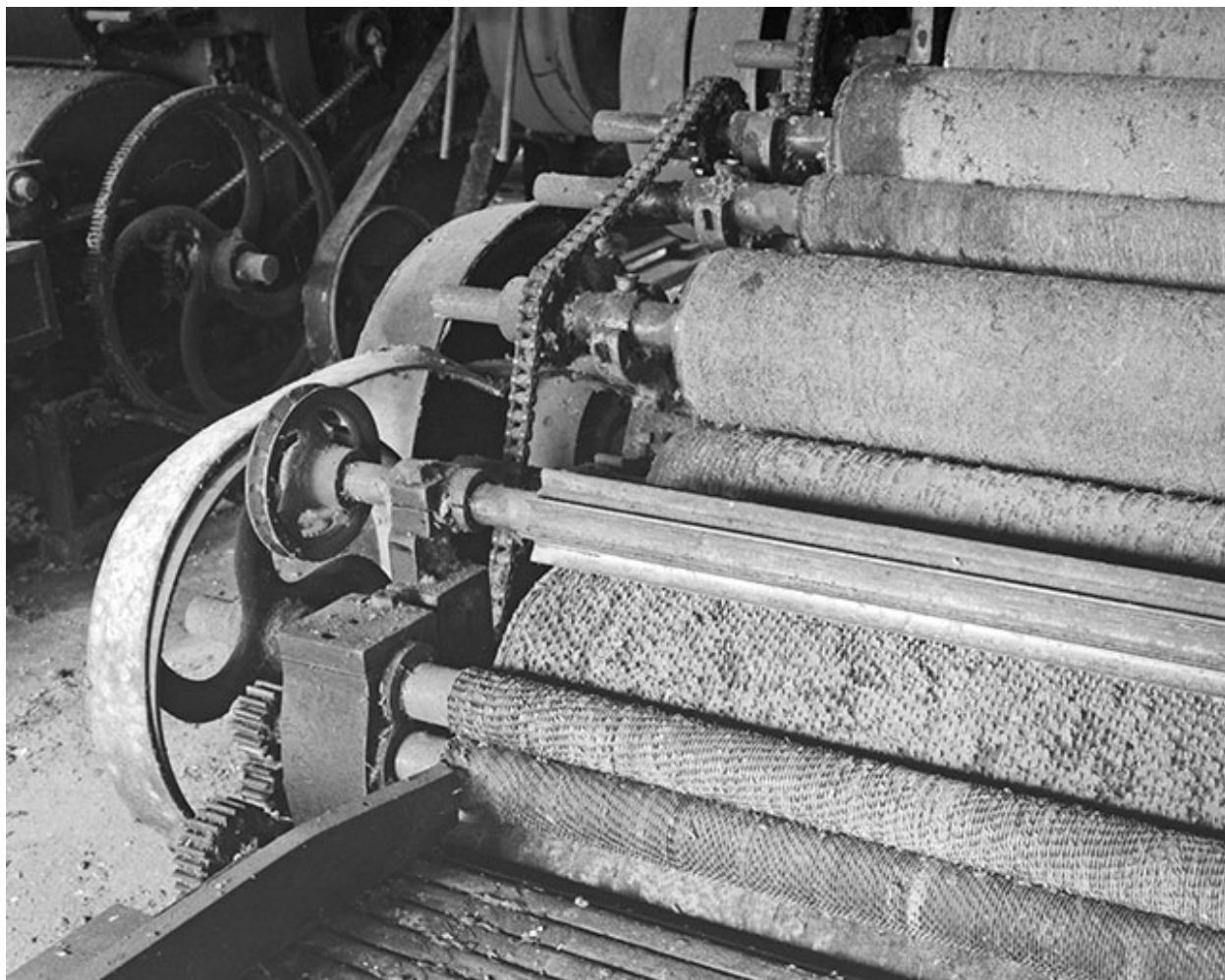
Détail du cylindre briseur. De gauche à droite, rouleaux alimentaires, cylindre briseur puis cylindres cardes de l'avant-train.
