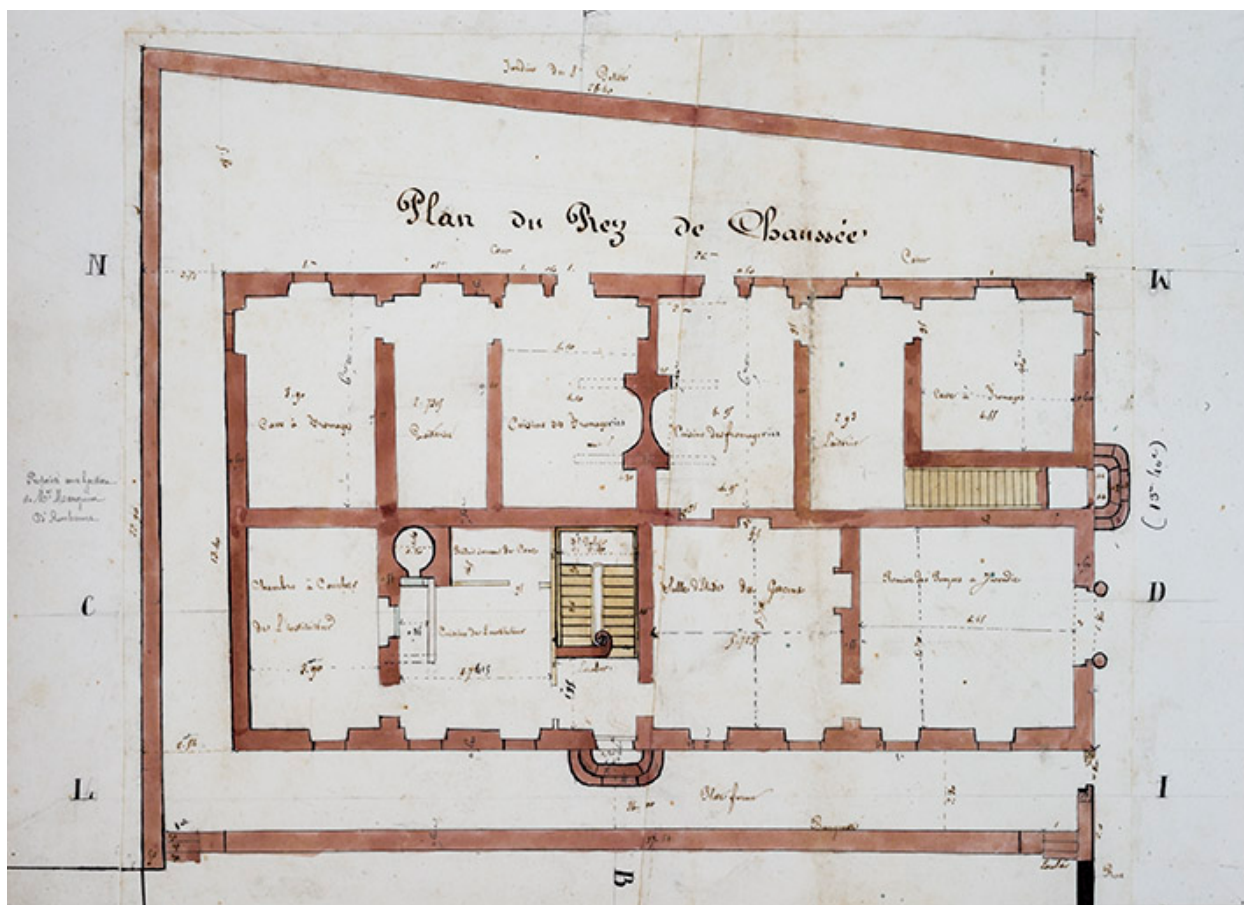
Plans, coupe et élévations du projet de construction d'une maison commune [...]. Plan du rez-de-chaussée, 1832.
