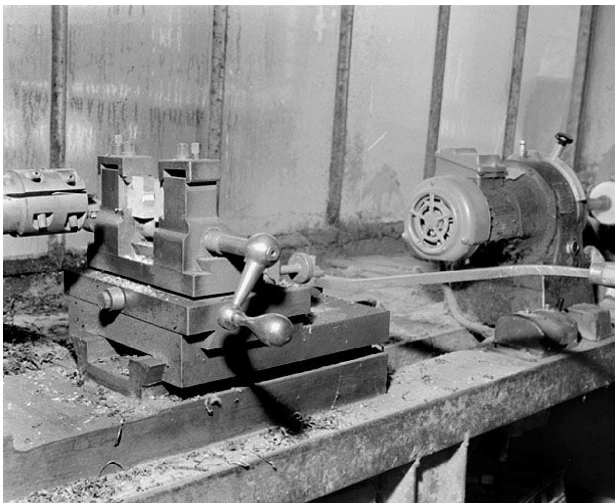
Mandrin porte-outils et chariot mobile.
