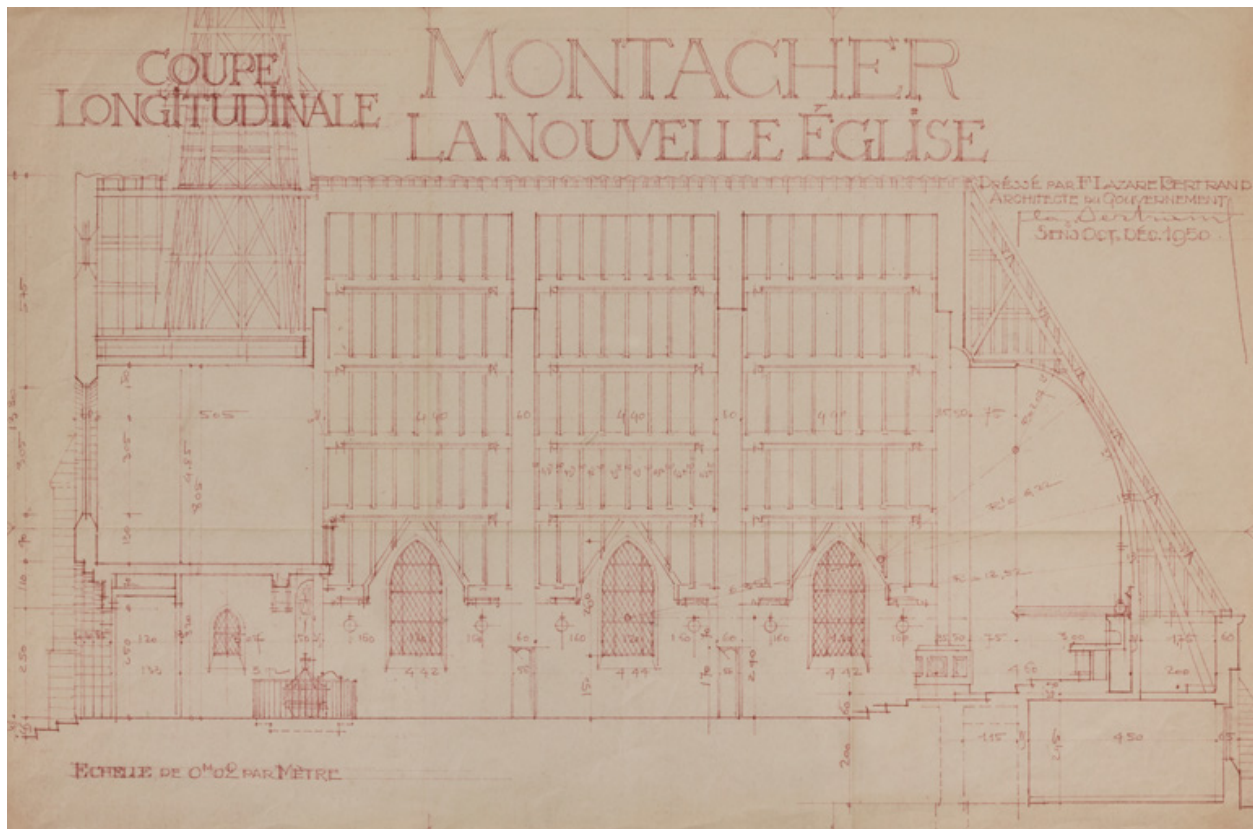
Coupe longitudinale de l'église, 1950.
