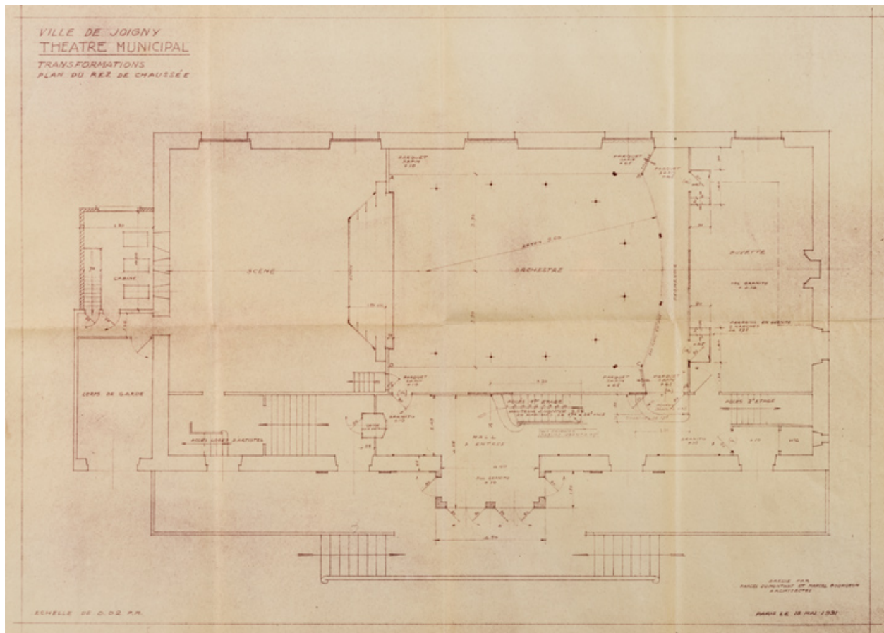
Théâtre municipal. Transformations. Plan du rez-de-chaussée. 18 mai 1931.
