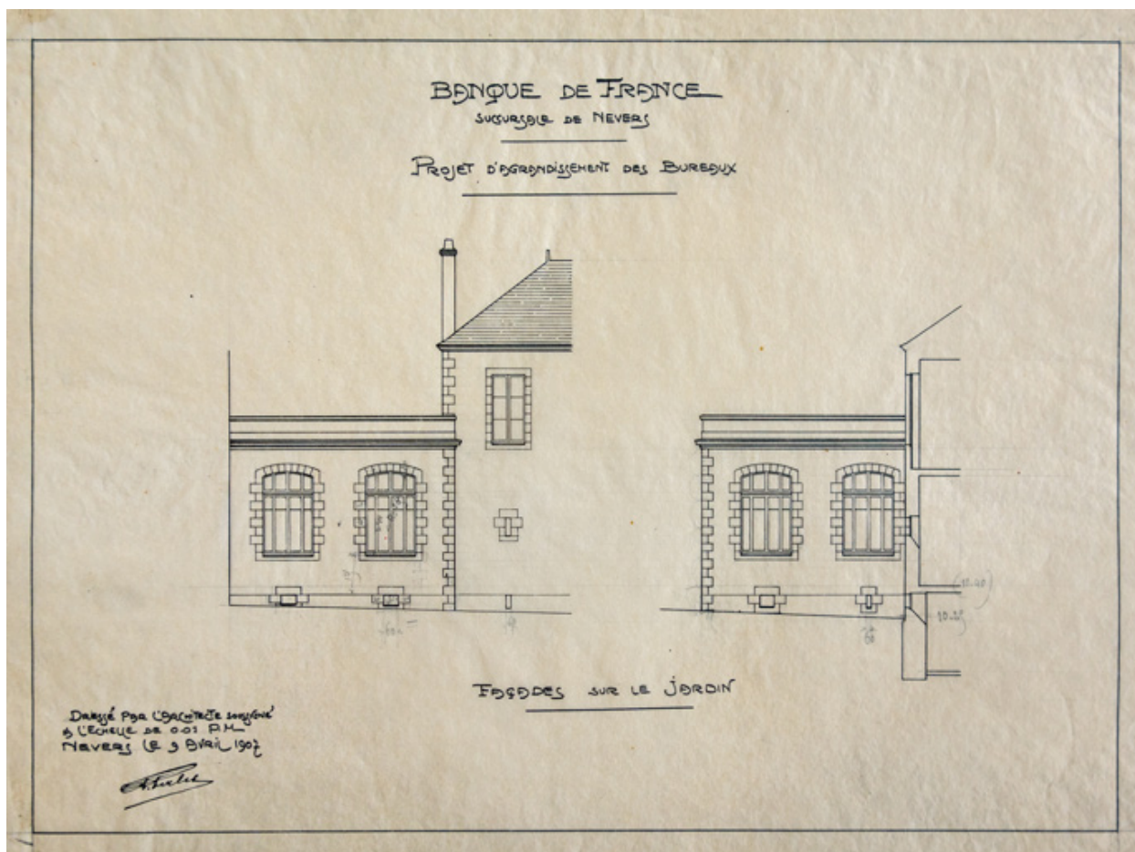
Façade sur le jardin, projet d'extension (9 avril 1907).
