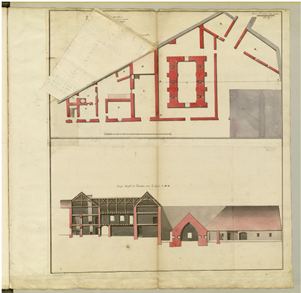
Fol. 15 Fort Saint-André-sur-Salins : plans, coupe, profil et élévation (magasin pour 60,000 milliers de poudre) - vue 2.
