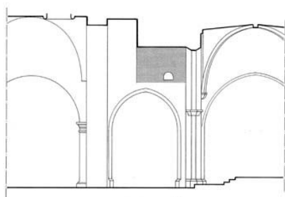
COUPE B.B'
