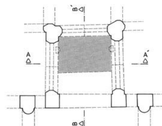
PLAN DE LA TRAVEE SOUS CLOCHER
