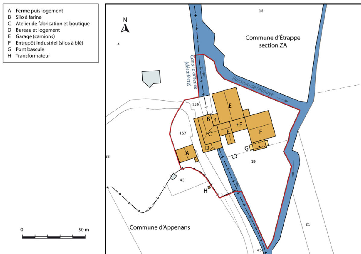
Plan-masse et de situation, extrait du plan cadastral, 2014, section B.
