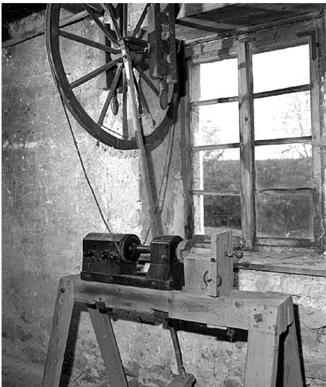
Tour à bois (tour à marchepied).
