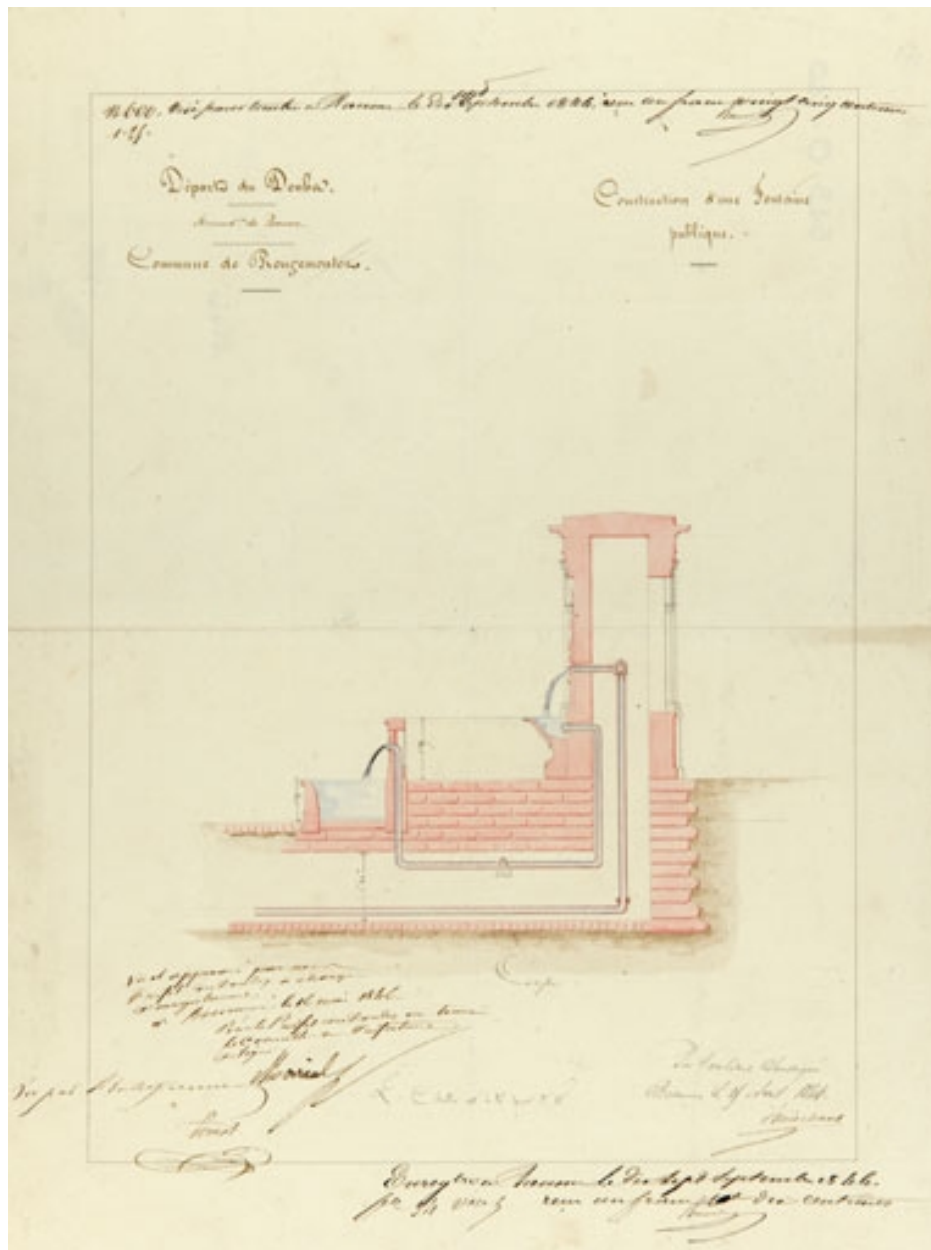
Construction d'une fontaine publique [coupe]. 1846.
