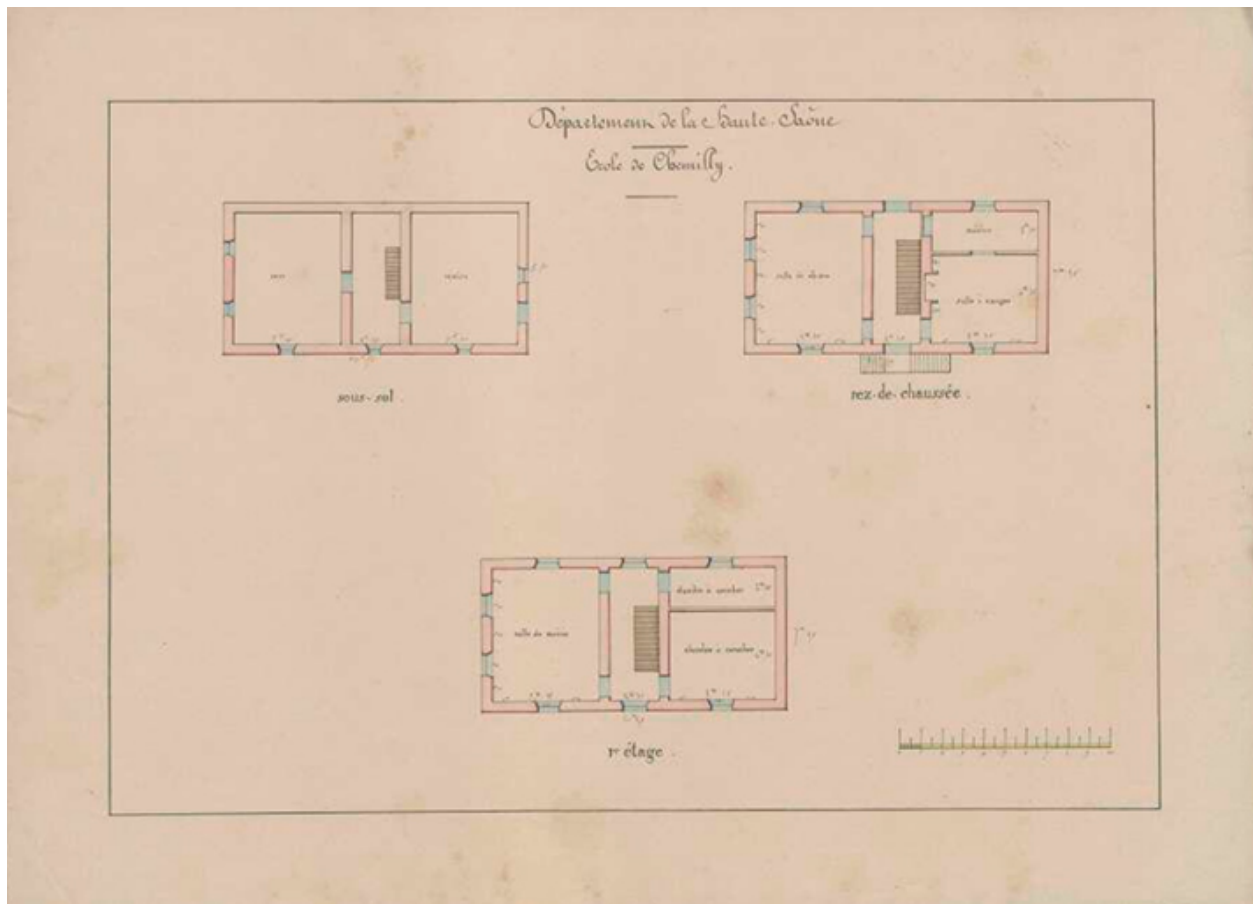
Plans en coupe du sous-sol, rez-de-chaussée et premier étage de l'école de Chemilly
