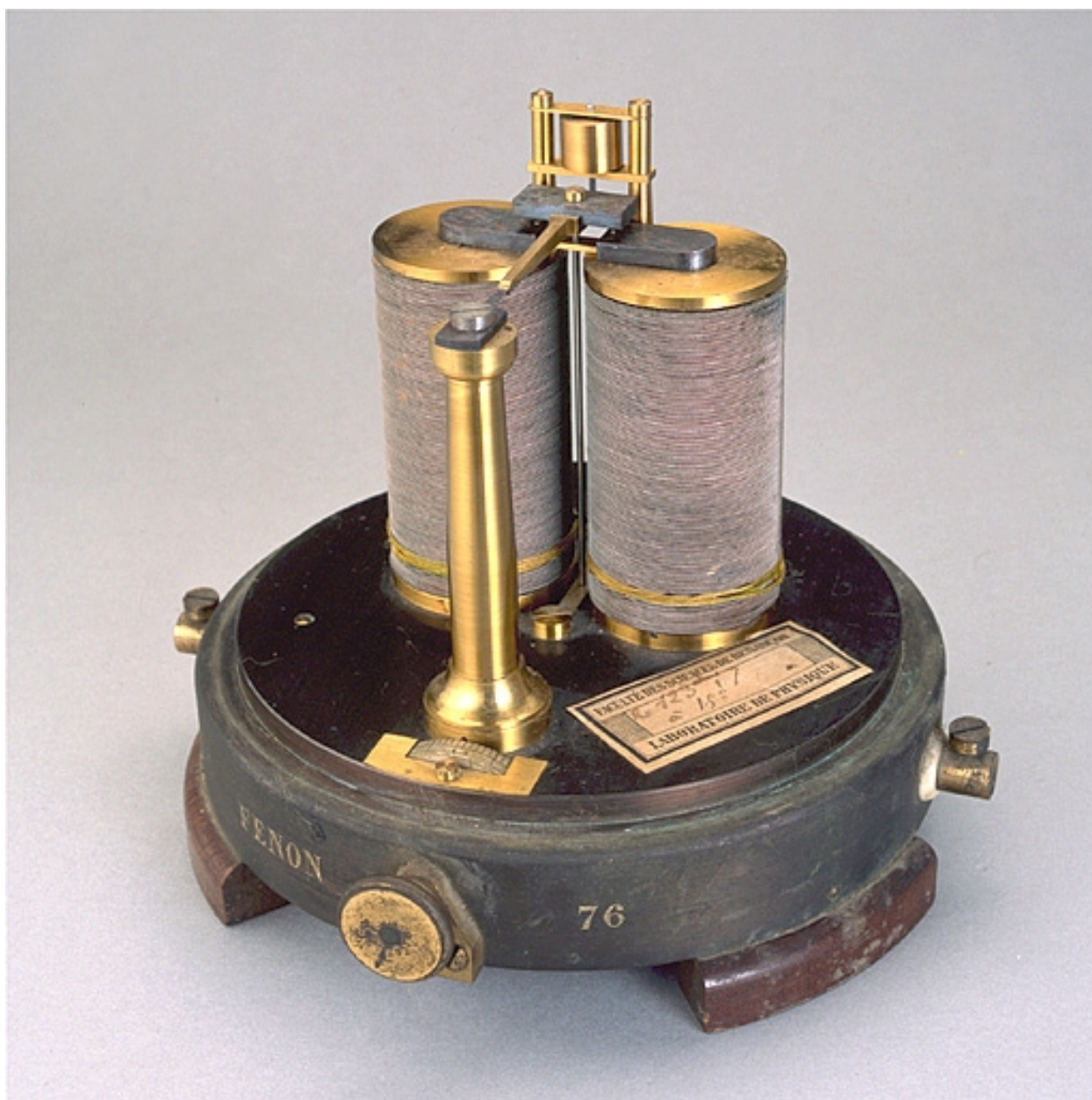
Le relais à deux bobines n° 76.
