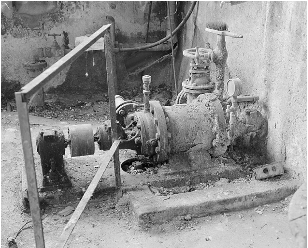
Pompe Sulzer, placée dans l'atelier de mécanique, permettant d'alimenter l'usine en eau depuis un réservoir placé à l'extérieur.
