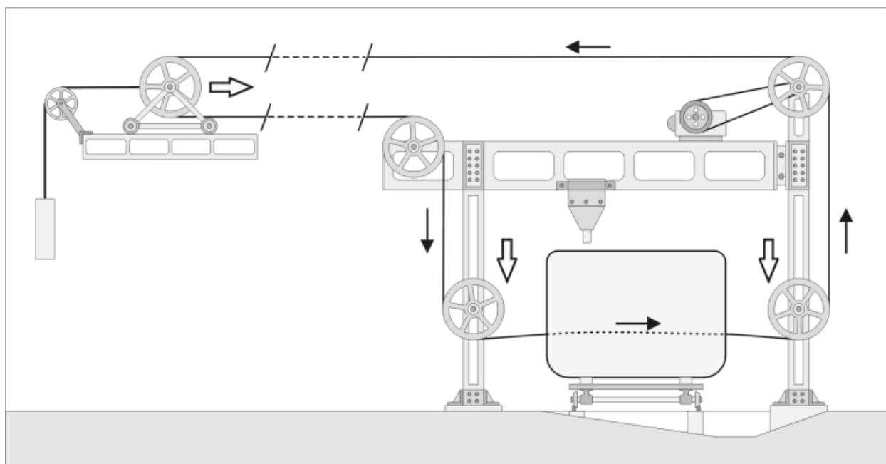
Schéma de fonctionnement d'une scie à fil hélicoïdal.
