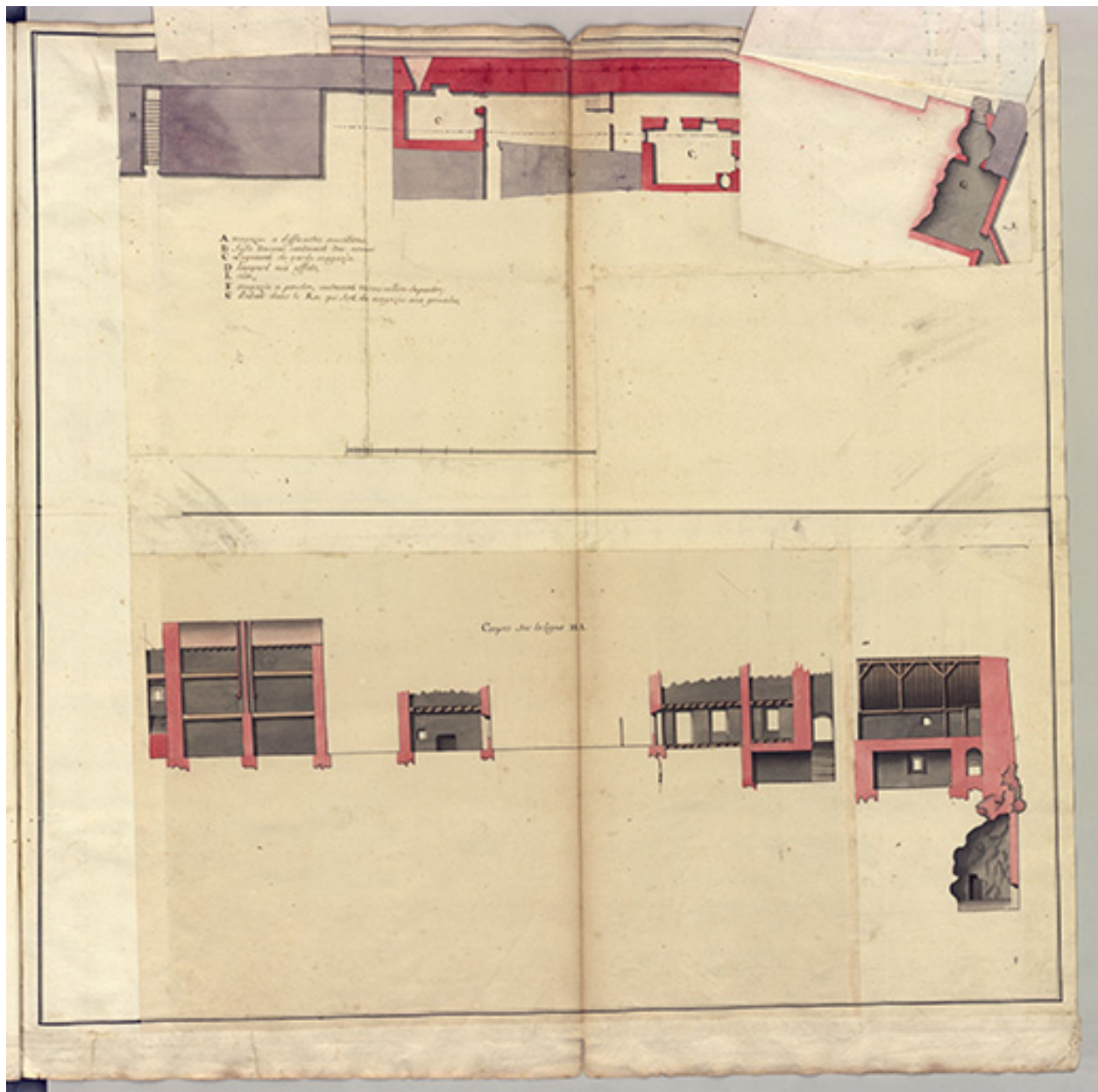
Fol. 16 Fort-Belin-sur-Salins : plans et coupes (magasin pour 12,000 milliers de poudre) - vue 3.
