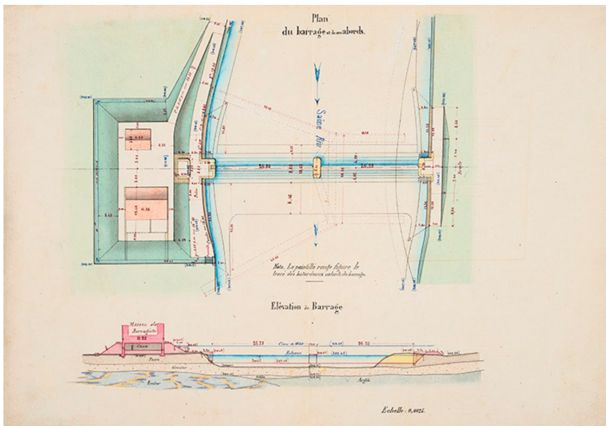
Canal de l'Est, projet des travaux de la dérivation de Port-sur-Saône - barrage mobile (1878) : détail du barrage et de ses abords.
